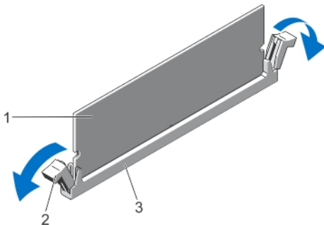
図 15. メモリモジュールの取り出し
