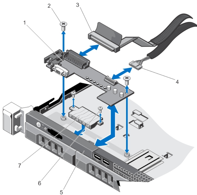
図 54. コントロールパネルモジュールの取り外しと取り付け—ケーブル接続式 3.5 インチハードドライブシステム
