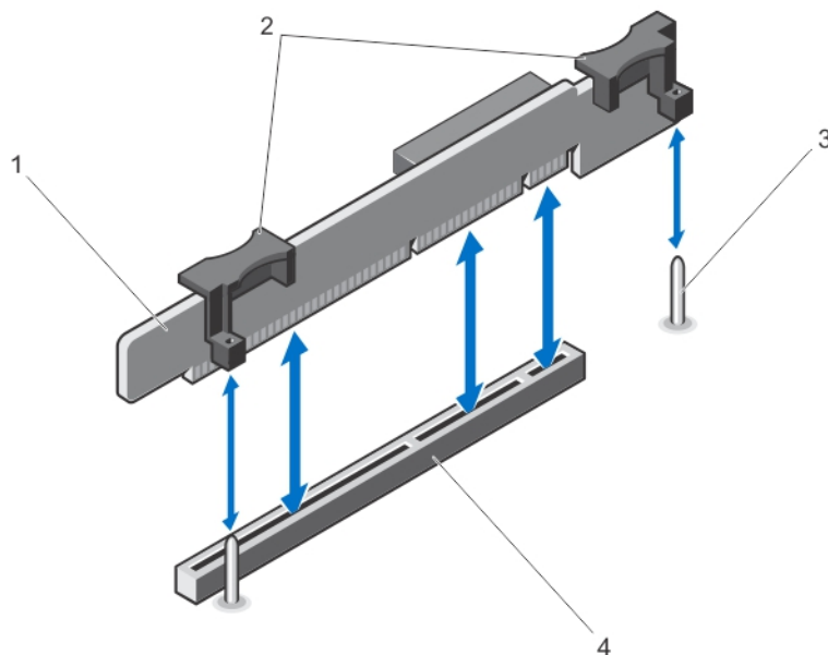
図 32. 拡張カードライザー 1 の取り外しと取り付け
