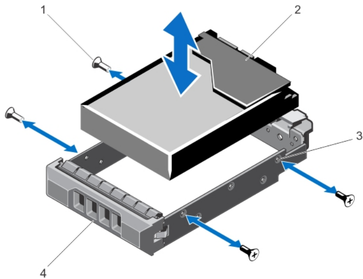
図 25. ケーブル接続式ハードドライブをハードドライブキャリアから取り外す/取り付ける方法
