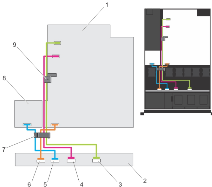
図 51. ケーブル接続図—ハードドライブ 8 台のバックプレーン
