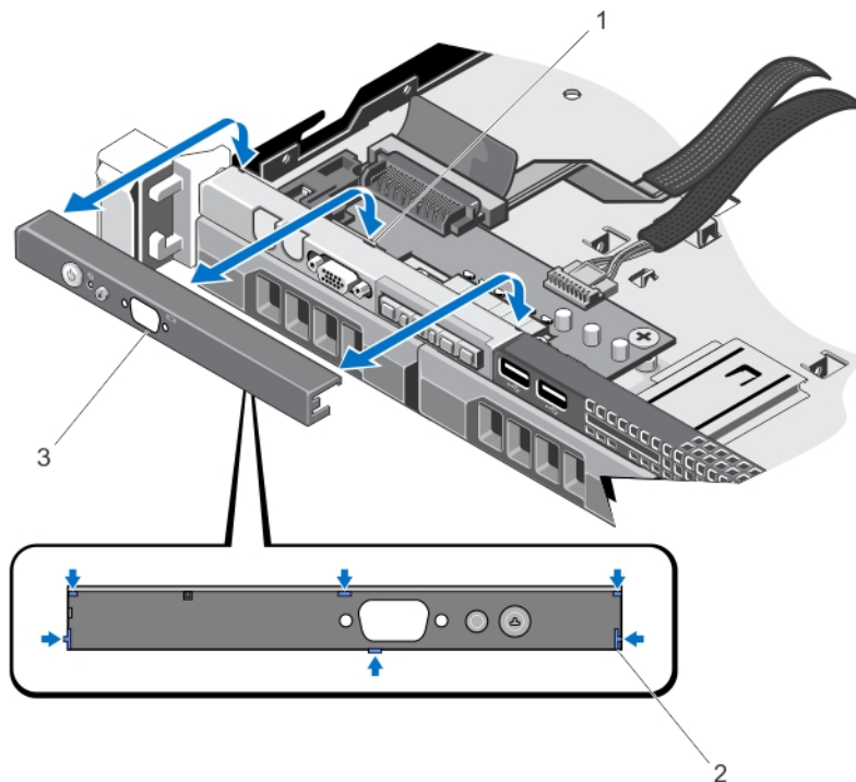
図 52. コントロールパネルの取り外しと取り付け — ハードドライブ 4 台のシステム
