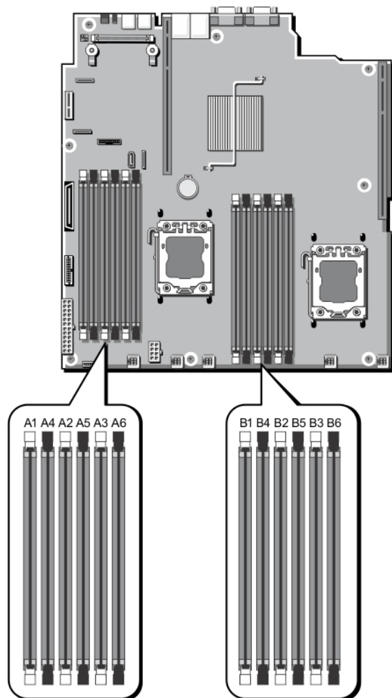
図 14. メモリソケットの位置
