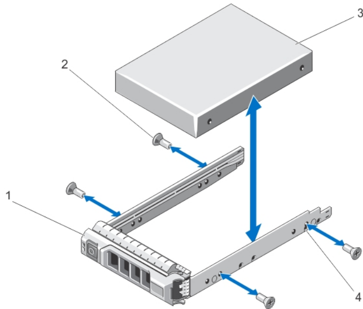
図 23. ホットスワップ対応ハードドライブのハードドライブキャリアからの取り外しと取り付け
