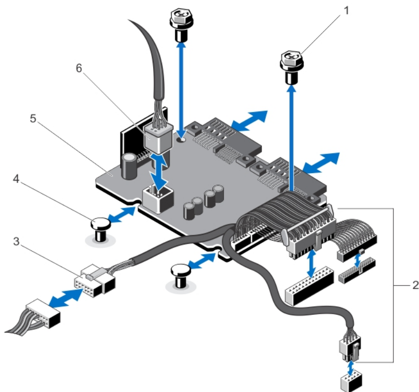
図 59. 配電基板の取り外しと取り付け
