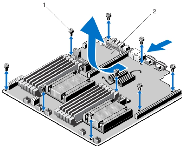
図 60. システム基板の取り外しと取り付け
