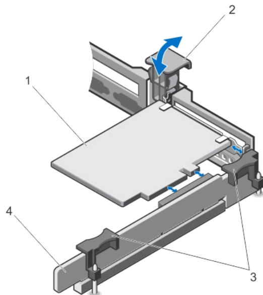
図 30. 拡張カードライザー 1 からの拡張カードの取り外しと取り付け
