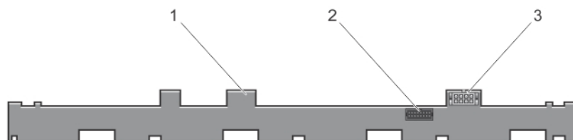
図 45. ハードドライブ 4 台のバックプレーンの背面図
