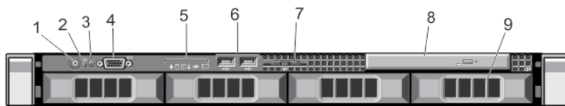
図 3. 前面パネルの機能とインジケータ — 3.5 インチケーブル接続式ハードドライブ 4 台のシステム
