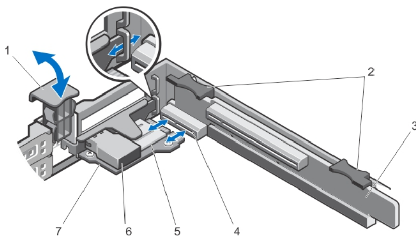
図 34. iDRAC ポートカードの取り外しと取り付け
