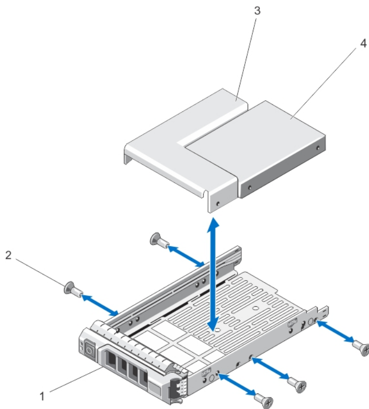
図 24.2.5 インチホットスワップ対応ハードドライブが入ったハードドライブアダプタを3.5インチハードドライブキャリアから取り外す/取り付ける方法
