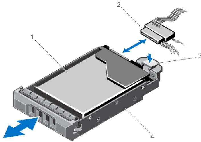
図 21. ケーブル接続式ハードドライブの取り外しと取り付け
