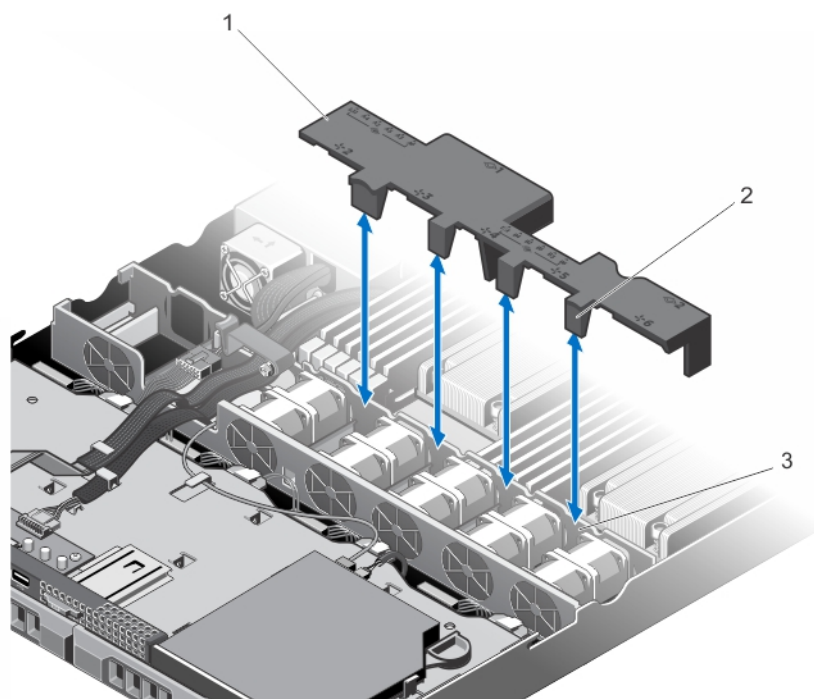
図 13. 冷却用エアフローカバーの取り外しと取り付け
