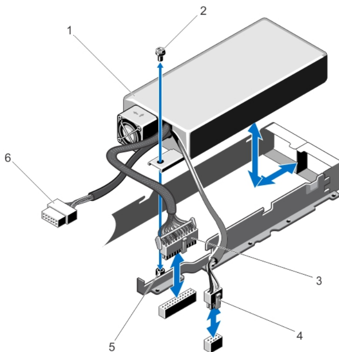
図 41. 非冗長電源ユニットの取り外しと取り付け
