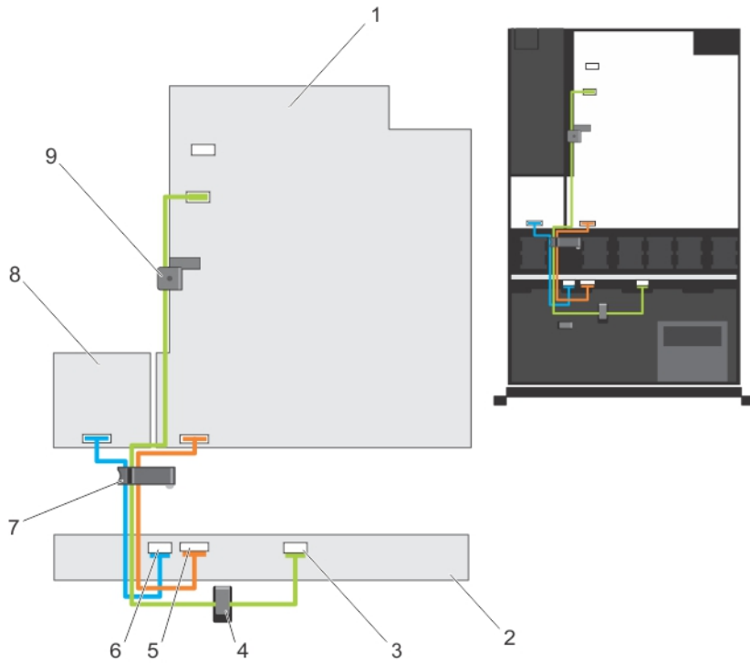
図 47. ケーブル接続図 — ハードドライブ 4 台のバックプレーン
