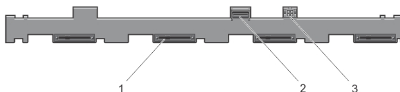
図 44. ハードドライブ 4 台のバックプレーンの正面図
