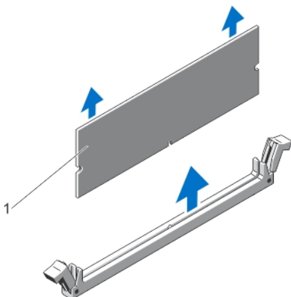
図 16. メモリモジュールの取り外し
