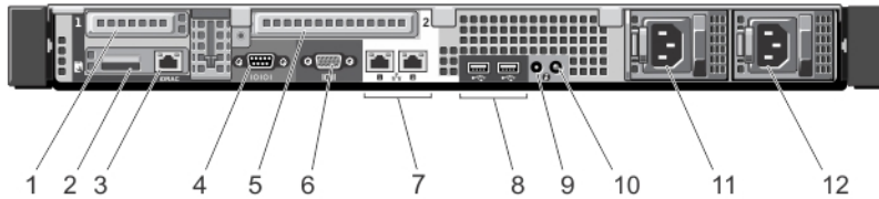
図 6. 背面パネルの機能とインジケータ
