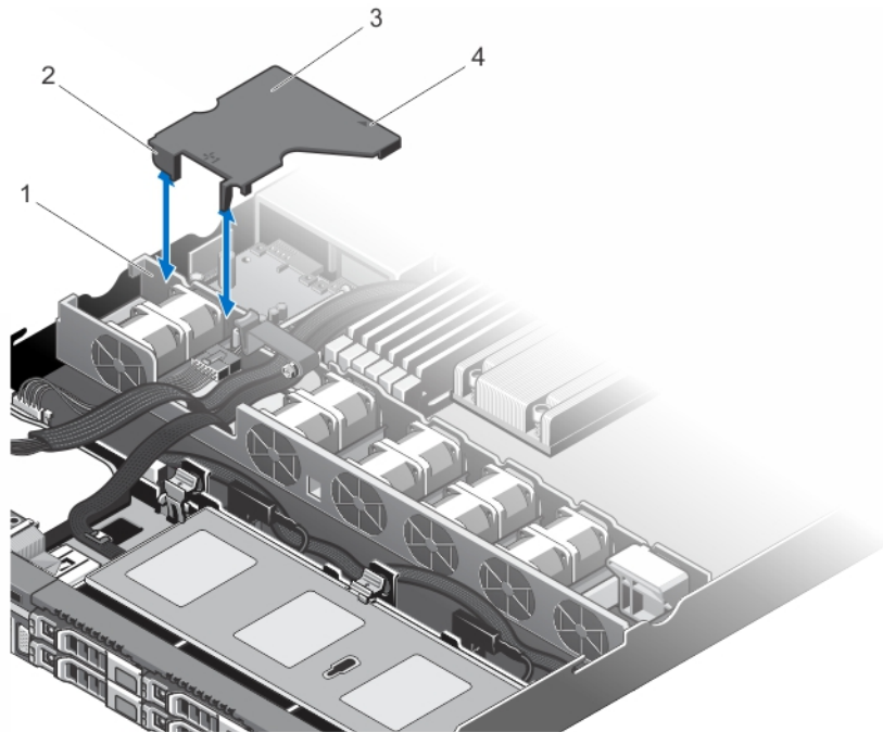
図 58. PDB エアフローカバーの取り外しと取り付け
