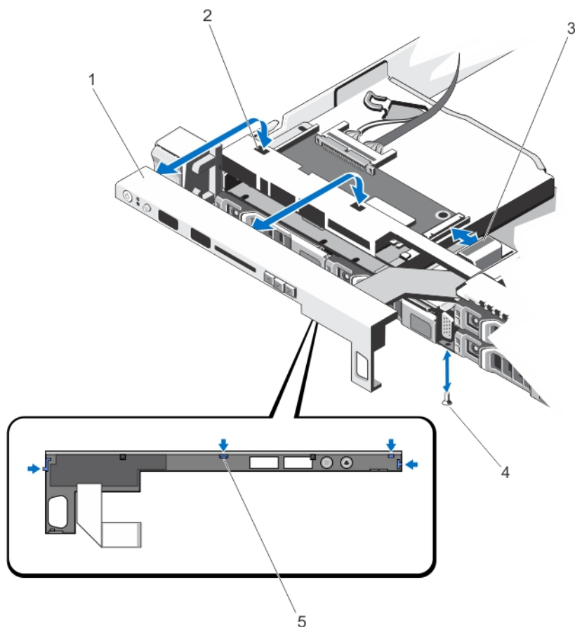
図 53. コントロールパネルの取り外しと取り付けーハードドライブ 8 台のシステム
