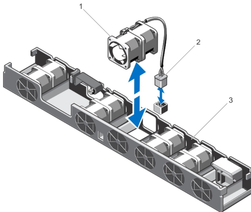
図 28. 冷却ファンの取り外しと取り付け
