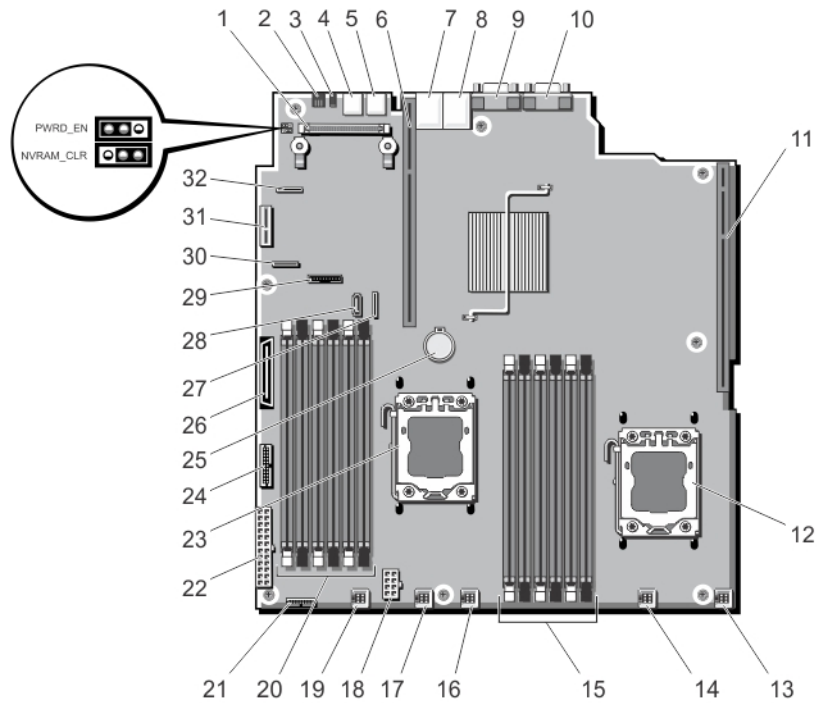
図 61. システム基板のジャンパとコネクタ
