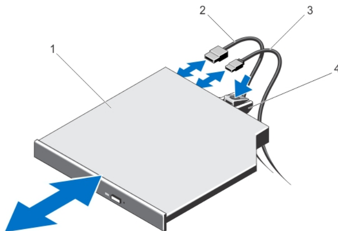
図 26. オプティカルドライブの取り外しと取り付け（ホットスワップ対応ハードドライブシステム）
