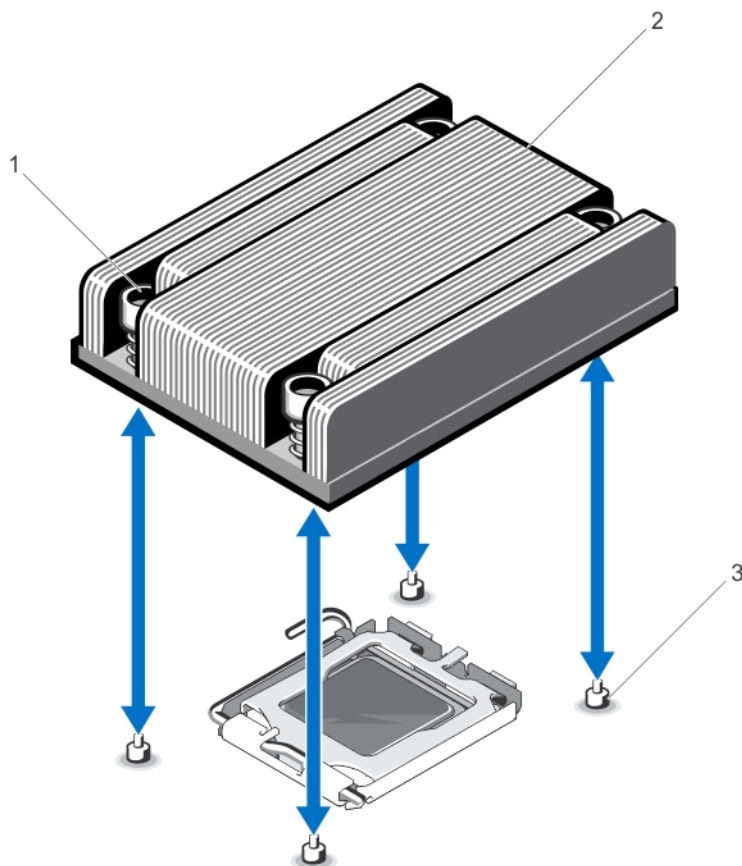
図 38. プロセッサヒートシンクの取り外しと取り付け
