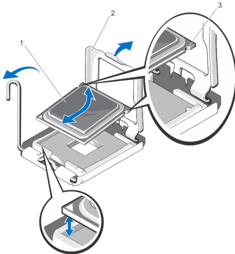
図 39. プロセッサの取り外しと取り付け
