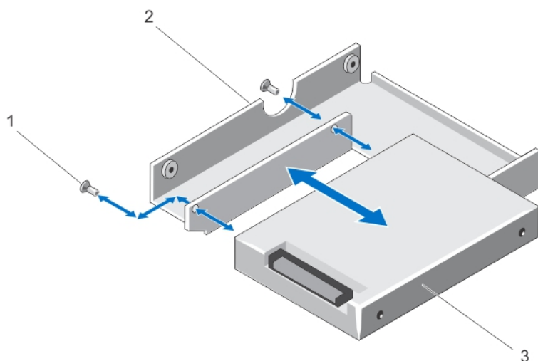
図 22. 2.5 インチハードドライブを 3.5 インチハードドライブアダプタから取り外す/取り付ける方法
